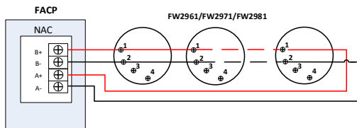
(d) Addressable – Class A with MA panel
